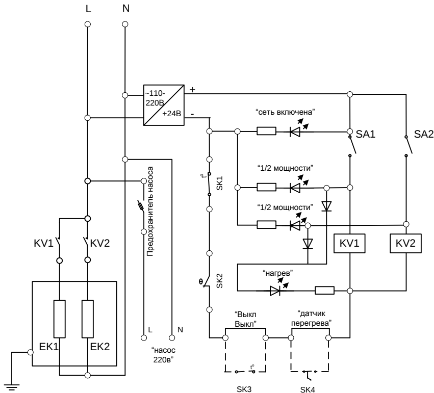
Рис.4 Схема электрическая принципиальная электронагревателя.
