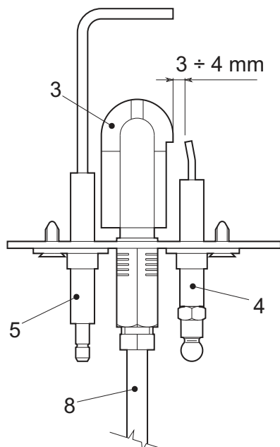
fig. 8 - Brûleur pilote
