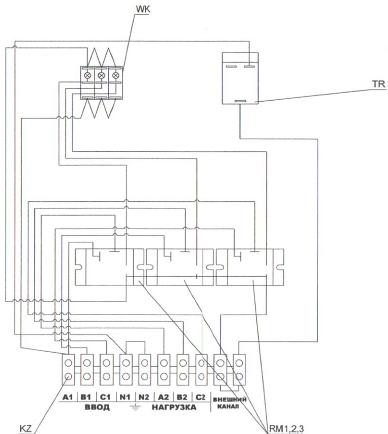
Рис.2 Схема монтажная.
