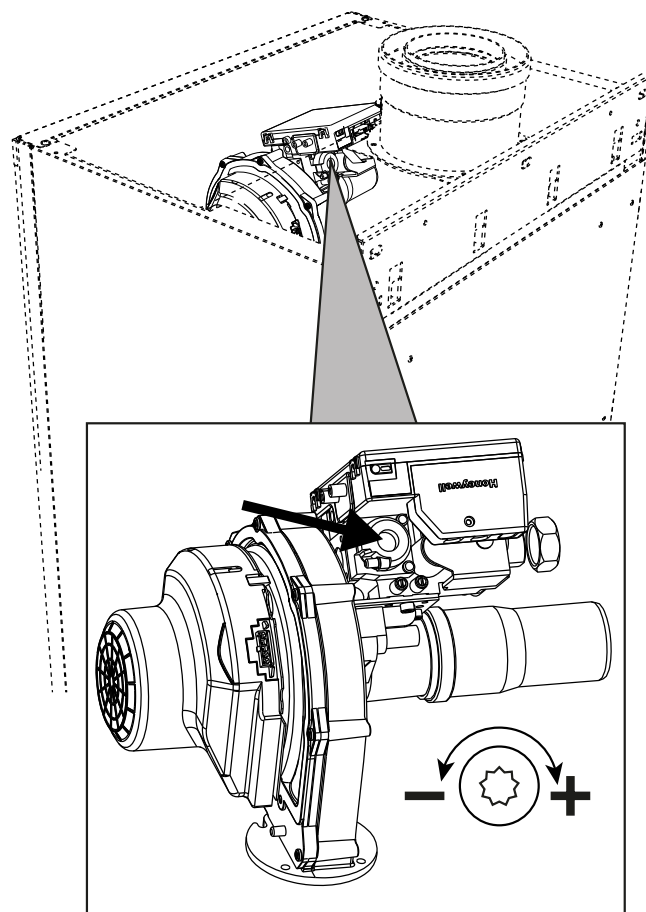
fig. 74 - Regolazione minima modelli W 60 e W 80
