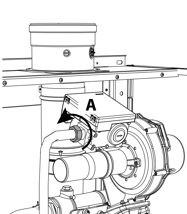
fig. 64- Modelos W 60 y W 80
