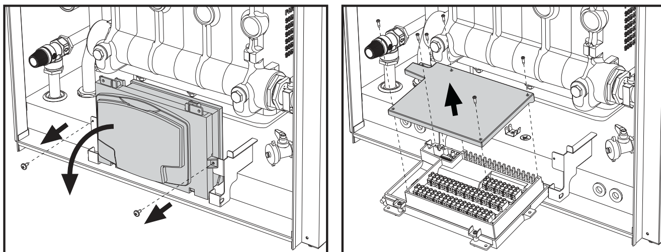
fig. 55- Regleta eléctrica
