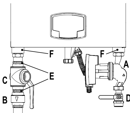
fig. 37- Caldera con kits instalados
