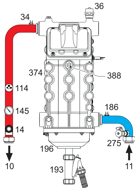
fig. 86- Circuitul hidraulic
