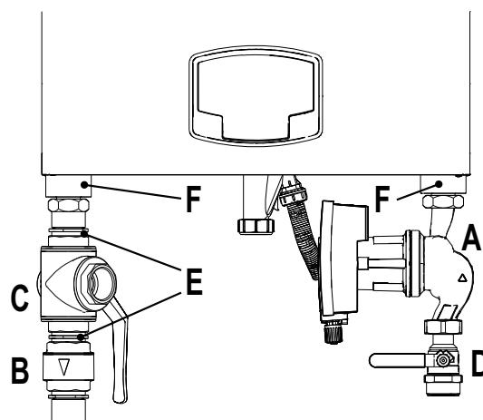
fig. 37- Chaudière avec les kits installés
