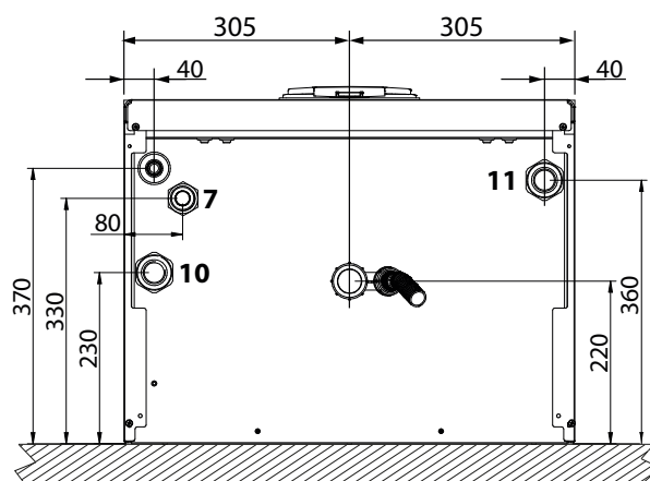
wygląd 82- Widok z góry
