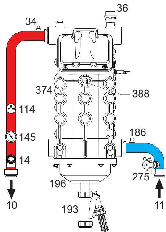
fig. 86- Circuito hidráulico
