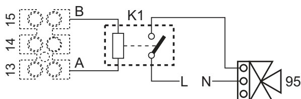
wygląd 89- Podłączenie zaworu 3-drożnego z 2 żyłami
