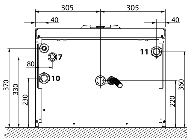
fig. 82- Vedere de sus
