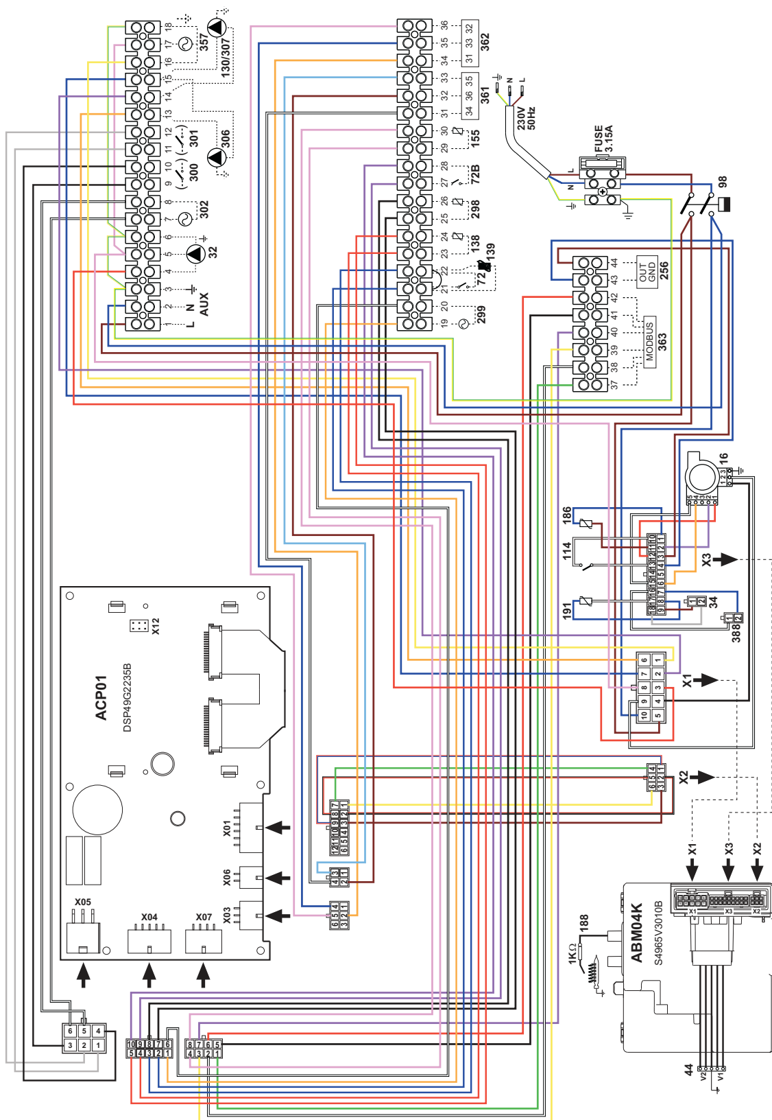
fig. 92- Esquema eléctrico modelos FORCE W 60 y FORCE W 80
