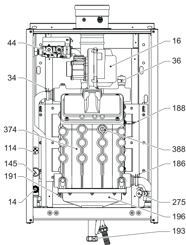
fig. 84- Vue générale mod. FORCE W 99 et FORCE W 120
