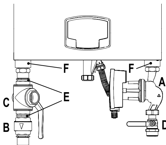
wygląd 37- Kocioł z zainstalowanymi zestawami
