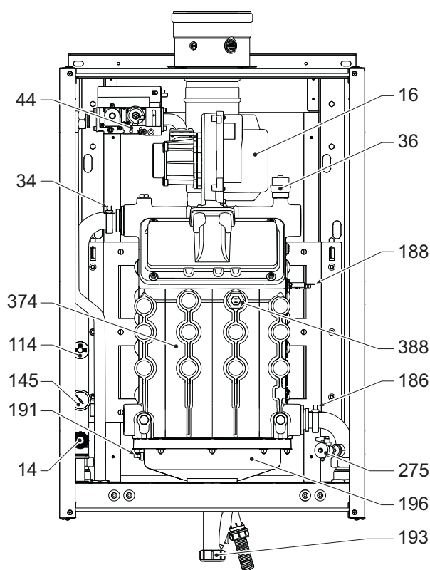
fig. 84 - Vista generale mod. FORCE W 99 e FORCE W 120
