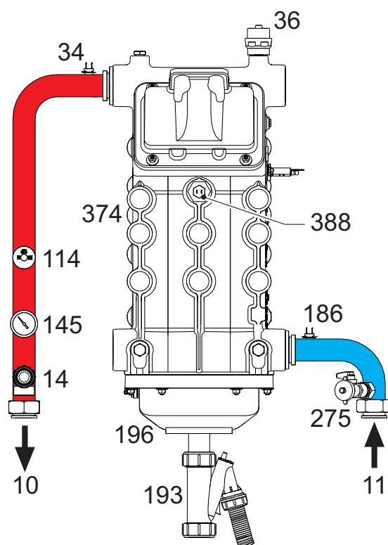
fig. 86 - Circuito idraulico
