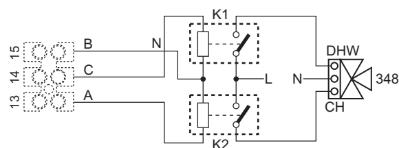
fig. 90- Raccordement de la vanne 3 voies à 3 fils
