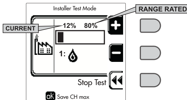
fig. 76- Modul TEST (exemplu putere de încălzire = 80%)
