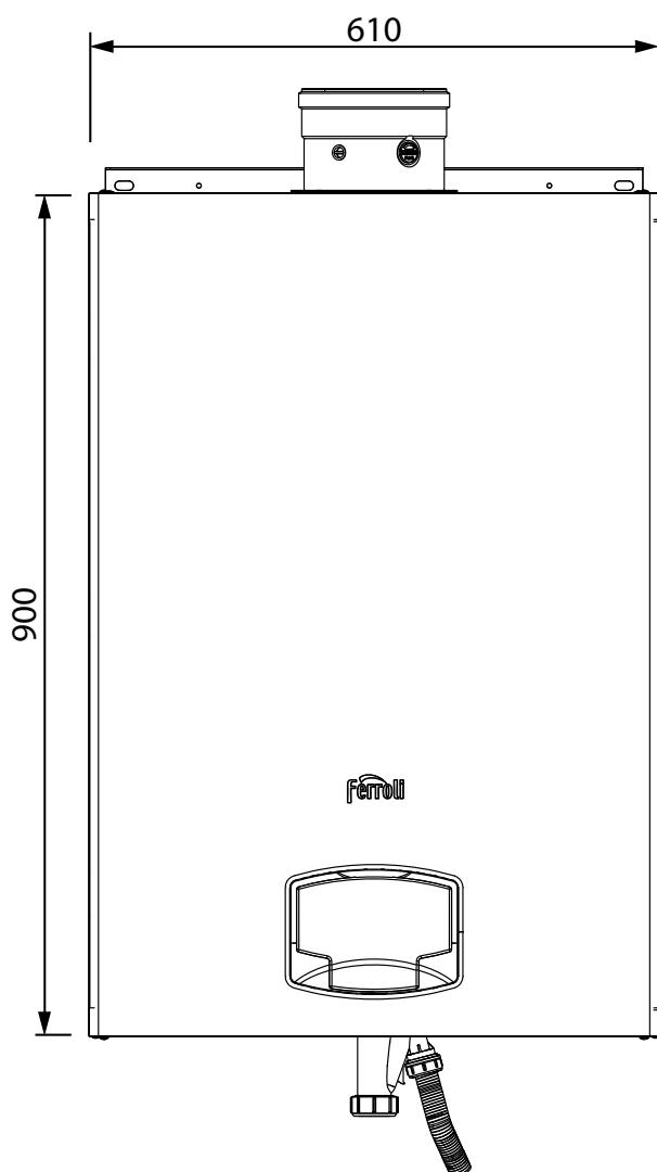
fig. 79- Vedere frontală
