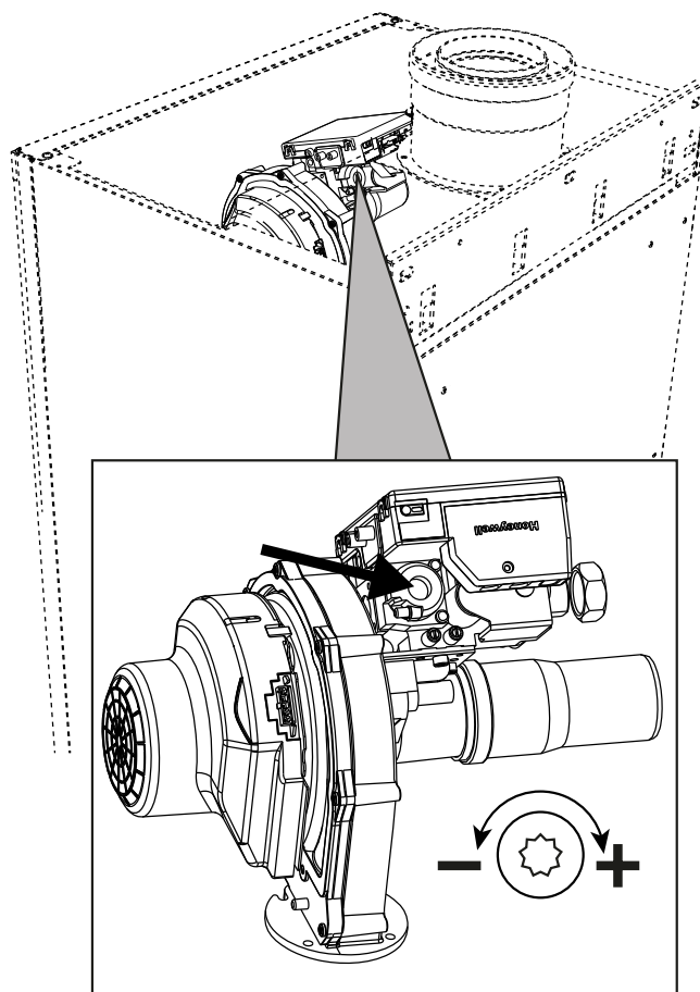
fig. 74- Réglage minimum modèles W 60 et W 80
