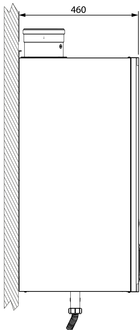
wygląd 80- Widok z boku
