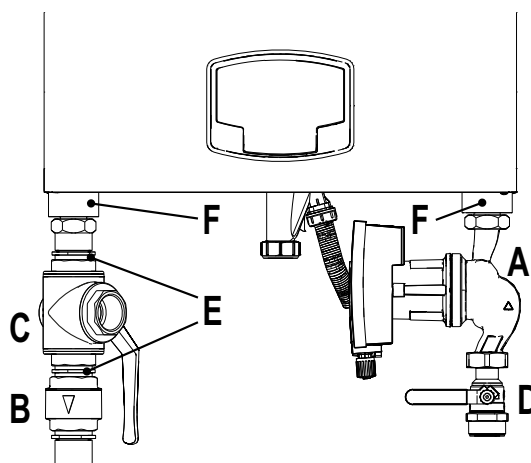
fig. 37 - Caldaia con i kit installati
