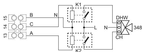
wygląd 90- Podłączenie zaworu 3-drożnego z 3 żyłami
