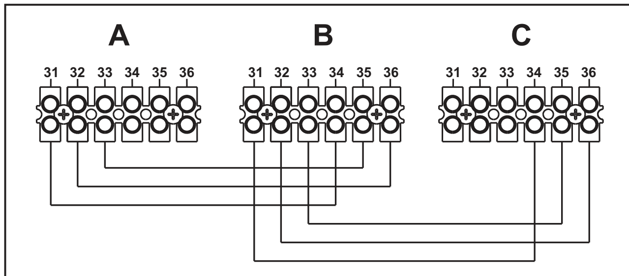
fig. 56 - Conexión en cascada
