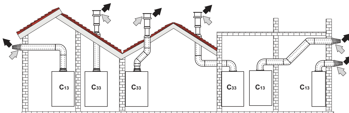
fig. 62- Exemples de raccordement avec tubes coaxiaux (→ = Air / → = Fumées)
