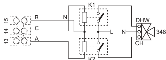
fig. 90- Racordarea valvei cu 3 căi cu 3 fire
