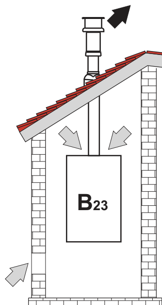
рис. 61- Примеры подключения (⇨ = Воздух/ ⇨ = Дымовые газы)
