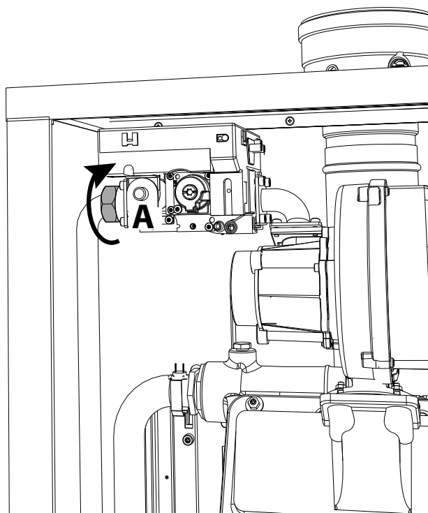
fig. 65- Modelos W 99, W 120 y W 150
