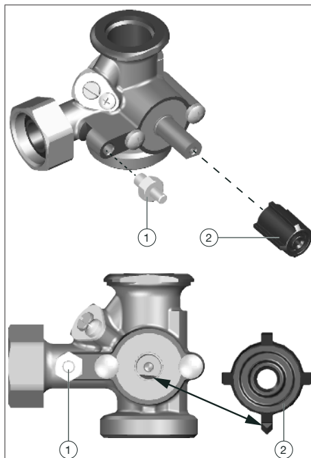
Abb. 3: Ausrichtung
