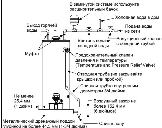
Рисунок 13 Установка водопровода
