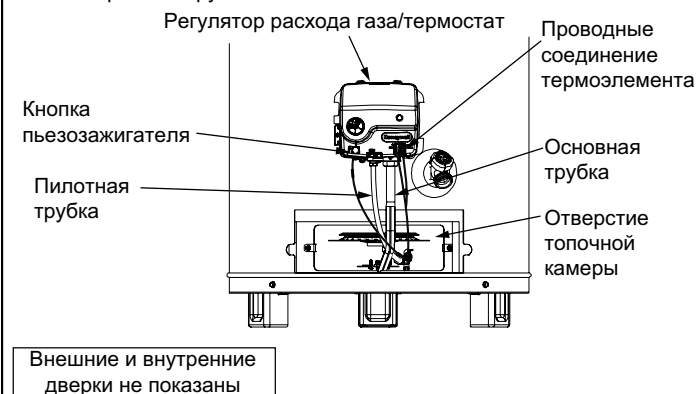
Рисунок 23 Снятие горелки с трубками
