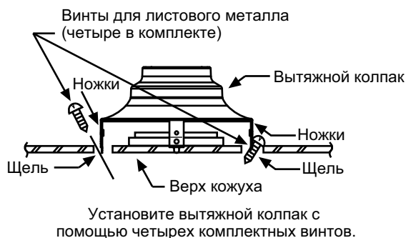
Рисунок 9 Установка вытяжного колпака
