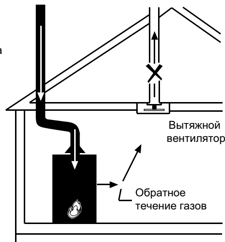
Рисунок 1Б Устройства, вызывающие движение воздуха
