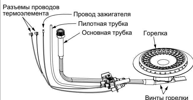
Рисунок 24 Горелка с трубками и проводами
