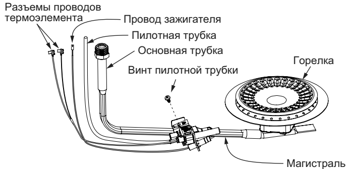
Рисунок 25 Винт пилотной трубки
