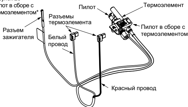
Рисунок 27 Связка трубок и проводов крупным планом
