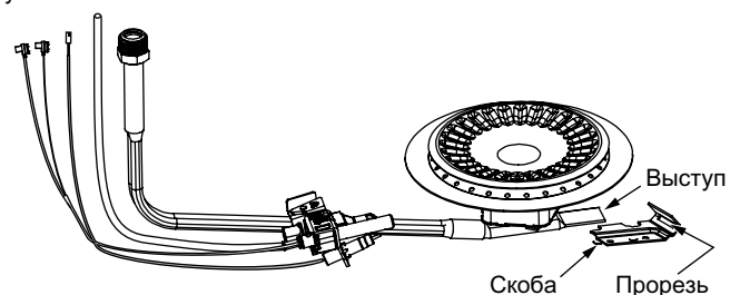
Рисунок 27 Связка трубок и проводов крупным планом
