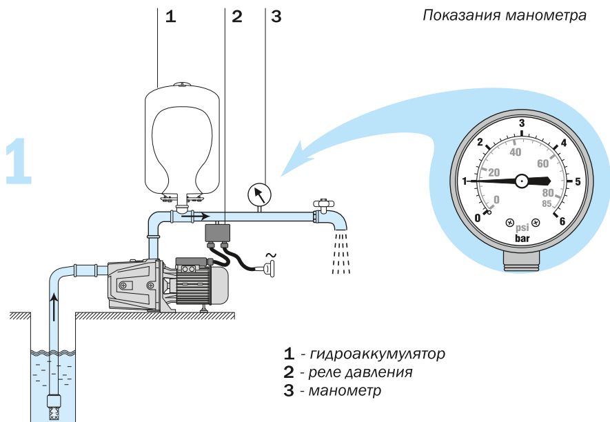
рис. 7. При запуске насосной станции и использовании водой насос включается и начинает качать воду потребителю.
