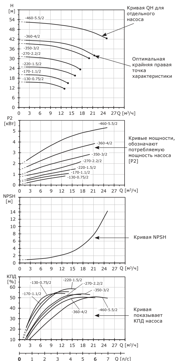
Рис. 12 Пример диаграммы рабочих характеристик насоса TPV
