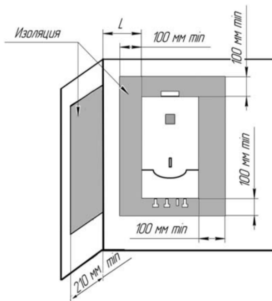
Рис. 3 Установка аппарата на трудносгораемых стенах.
