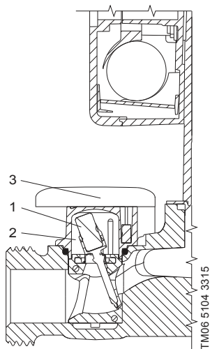
Рис. 2 Разрез внутреннего реле потока, UPA 15-120
