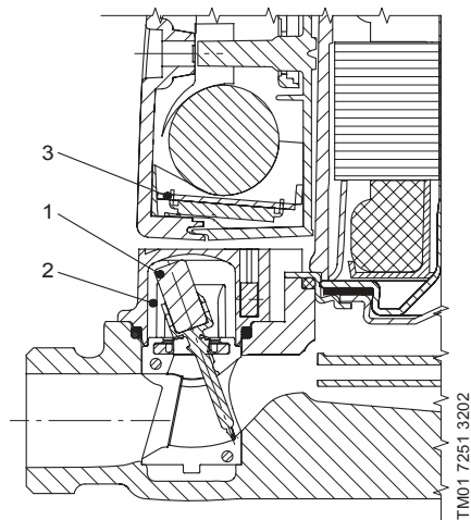
Рис. 1 Разрез внутреннего реле потока, UPA 15-90(N)
