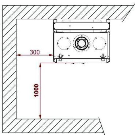
Рис. 3. Установка котла.
