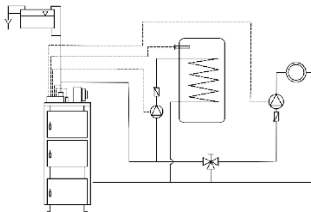
Рисунок 4 - Подключение с трехходовым клапаном и водонагревателем
