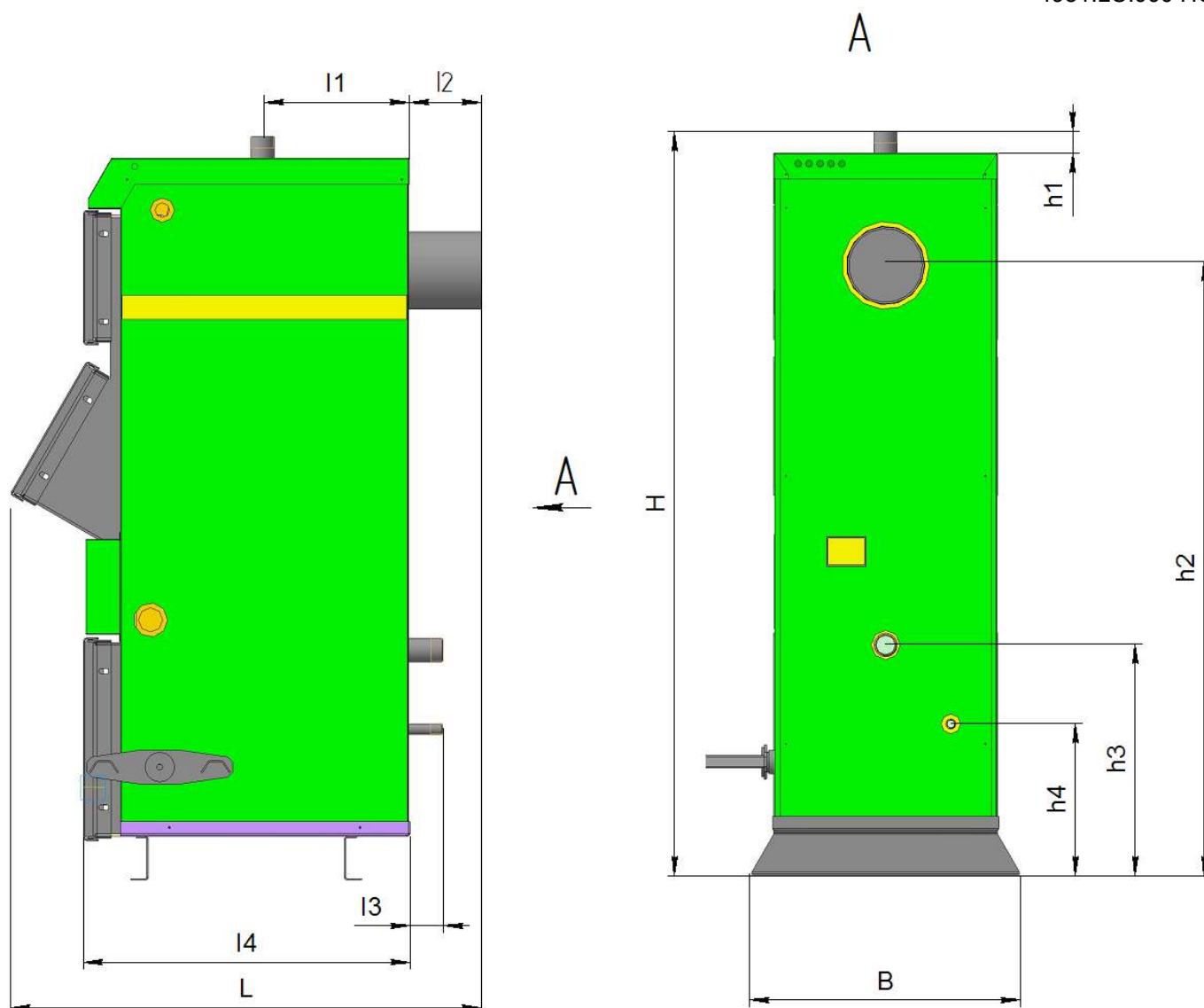
Рисунок 1 - Габаритные и присоединительные размеры Котлов моделей LC12-32
