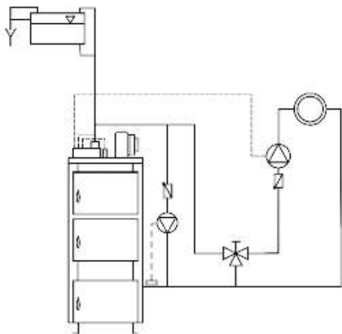
Рисунок 3 - Подключение с трехходовым краном
