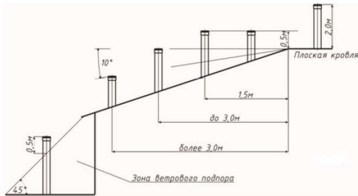
Рисунок 5 - Вылет трубы дымовой трубы в зависимости от конструкции кровли
