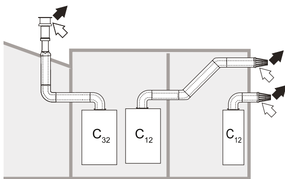
Рис. 16. Пример систем дымоудаления собранных с помощью коаксиальных труб. Белой стрелкой обозначен приток воздуха, черной стрелкой отвод продуктов сгорания.
