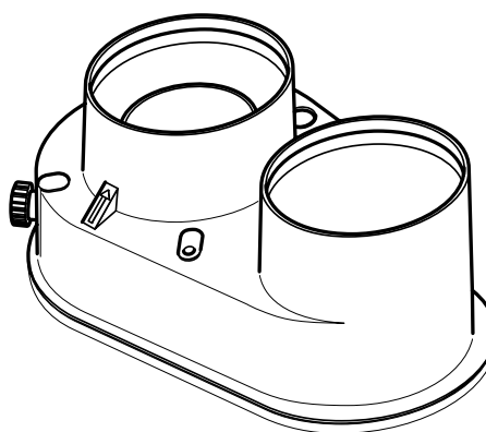
Рис. 13. Переходник с коаксиальной системы дымоудаления Ø 60/100 мм на раздельную Ø 80/80 мм.
