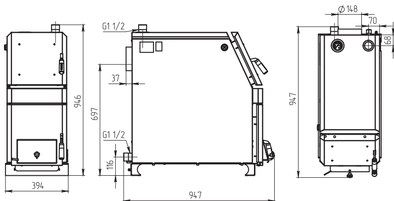
Рис.4 Габаритные размеры котла ZOTA Forest 31 кВт
