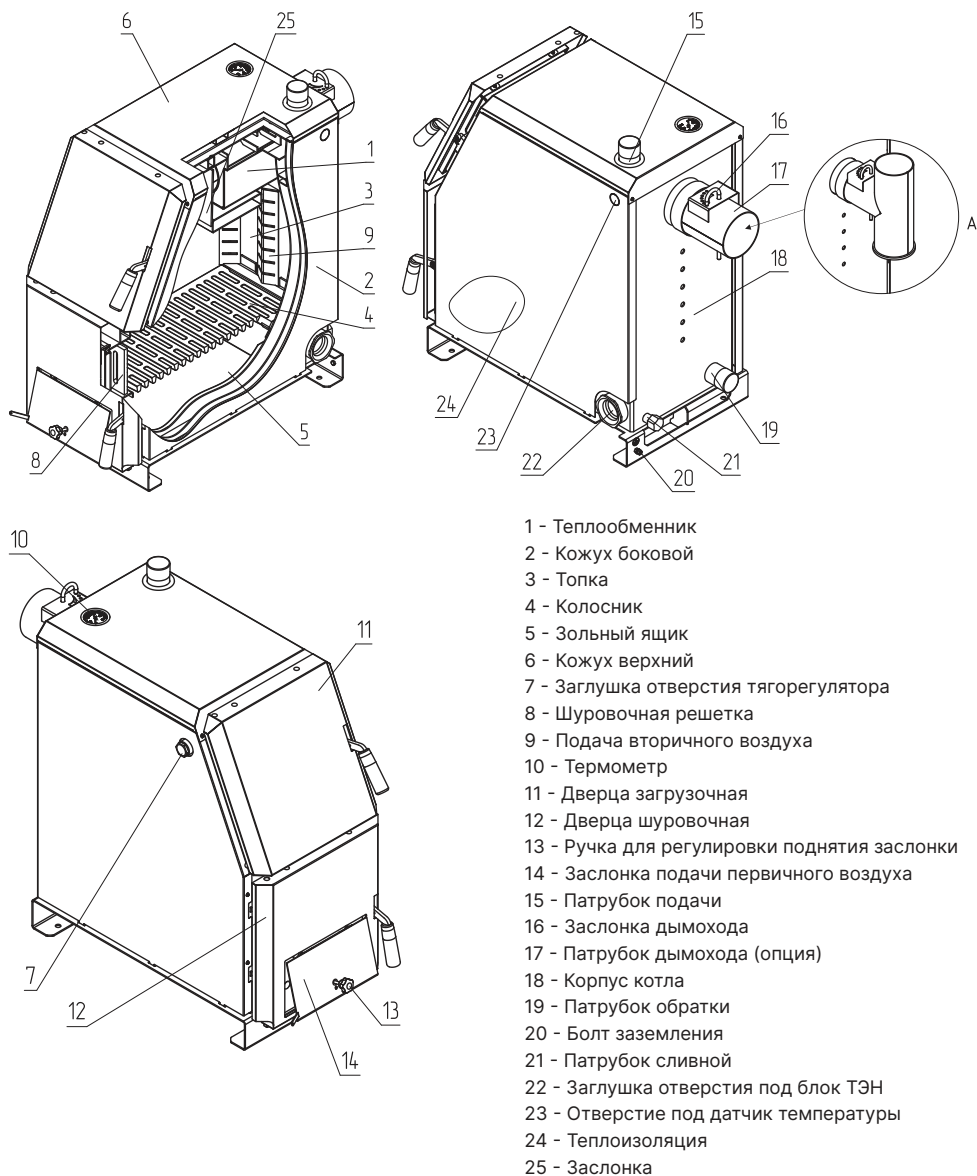
Рис.1 Устройство котла ZOTA Forest
