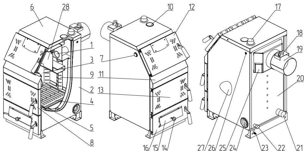
Рис.1 Устройство котла ZOTA Тополь-М
