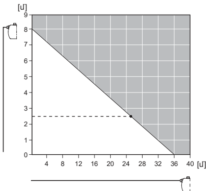
Նկար 9 Ներմղման խողովակաշարի առավելագույն երկարությունը (հորիզոնական առանցք) կախված ներմղման բարձրությունից (ուղղաձիգ առանցք)
