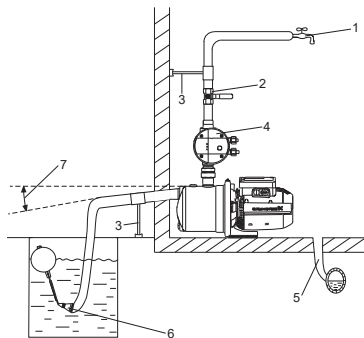
10-сүр. JP соркысмасын куроо мисалы, бактан/резервуардан сордуруу
