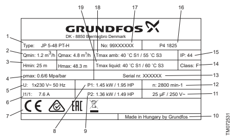
3-сүр. JP соркысмаларынын фирмалык көрнөкчөсү
