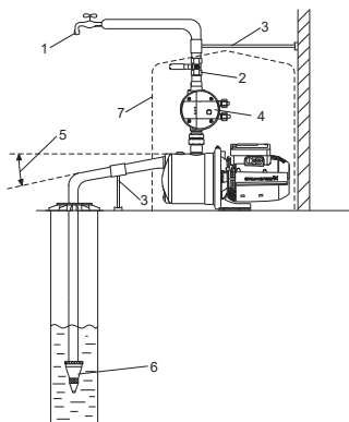
11-сүр. JP соркысмасын куроо мисалы, сууну скважинадан чогултуу
