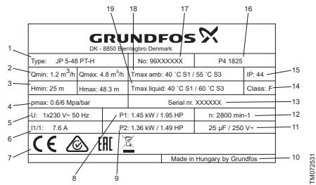
3-сур. JP сорғыларының фирмалық тақтайшасы
