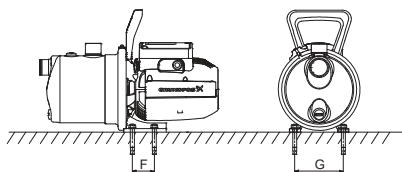
5-сур. JP сорғысының іргетасы
