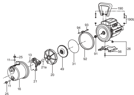
2-сүр. JP соркысмасын деталдаштыруу
