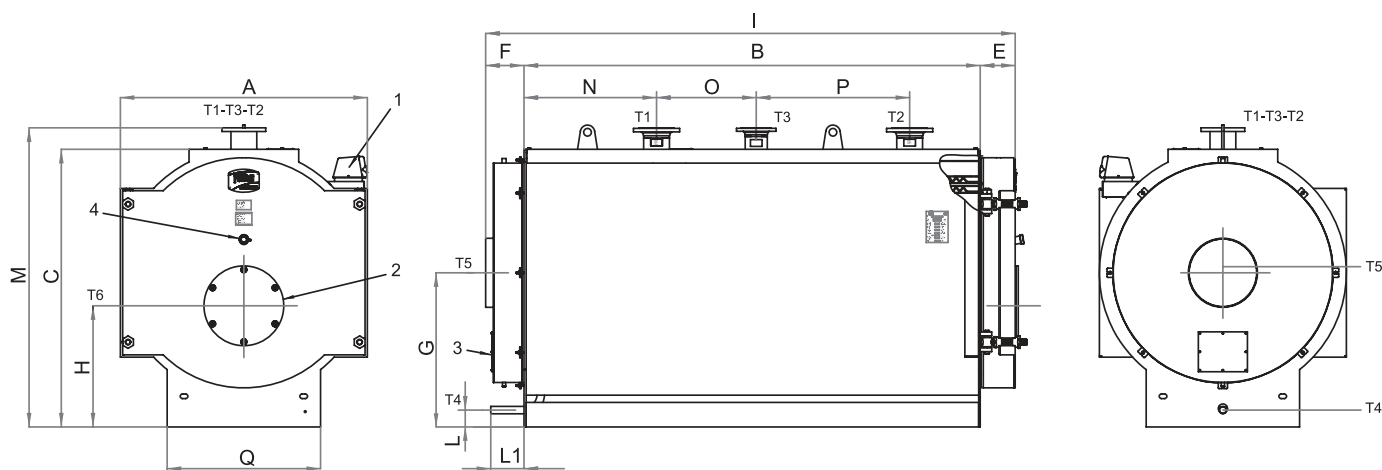
рис. 4 - RSW 2360N+6000N
