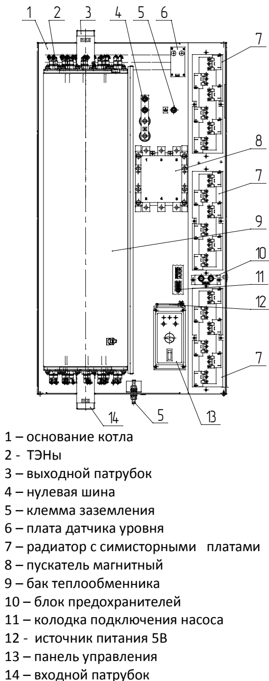
Рисунок 1. Устройство отопителя РЭКО 70П, 100П
