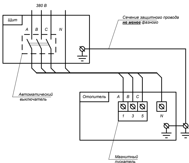
Рисунок 3. Подключение отопителя к электрической, трехфазной(380В), сети
