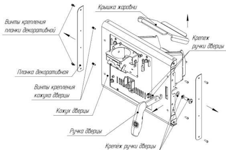
Рисунок 17 - Демонтаж кожуха двери, ручки и крышки жаровни
