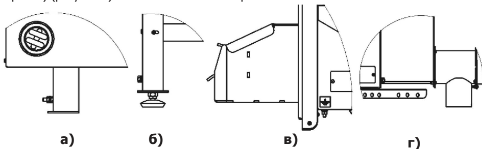
Рисунок 8 - Размещение болта заземления. (а) ножка котла, (б) бункер напольный, (в) горелочное устройство, (г) бункер котельный.
