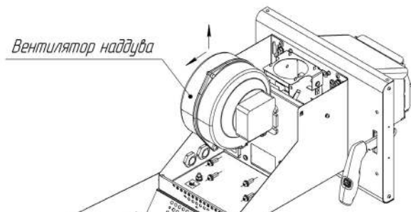
Рисунок 14 - Замена вентилятора надува
