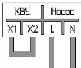
Рисунок 9 Схема подключения насоса и управляющего контакта
