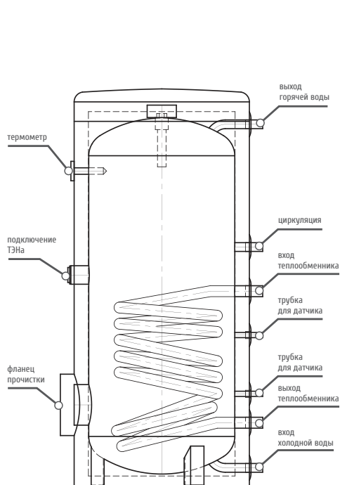
БОЙЛЕРЫ С ОДНИМ ТЕПЛООБМЕННИКОМ
