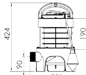
SANIPUMP® Vortex
