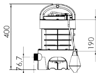
SANIPUMP® mit Zerkleinerungsschneidwerk
