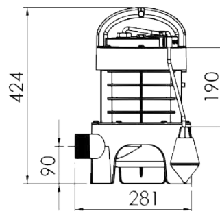
SANIPUMP® com Vortex
