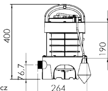
Rozdrabniacz SANIPUMP®
