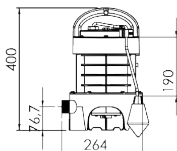
SANIPUMP® com trituração
