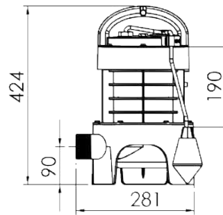
SANIPUMP® Vortex
