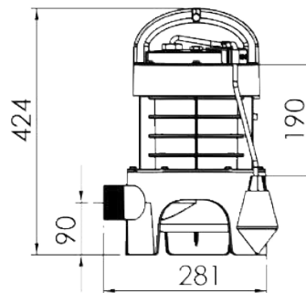
SANIPUMP® Vortex
