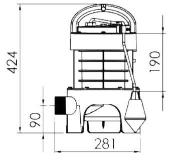
SANIPUMP® Vortex
