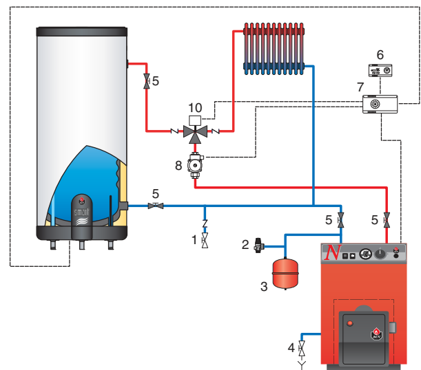
Бойлер с 3x-ходовым моторизированным клапаном. Вариант вертикального монтажа.
