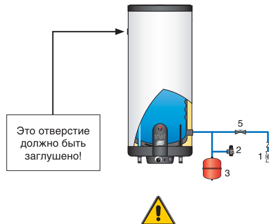
Бойлер SLE W , используемый как электрический нагреватель санитарной воды
