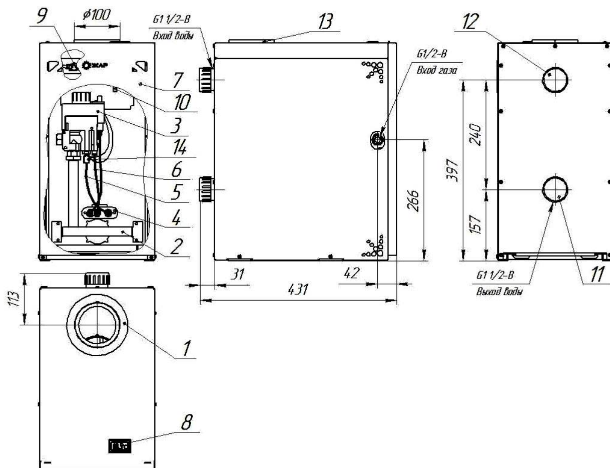
Рисунок 2 – котел AXIS-05
