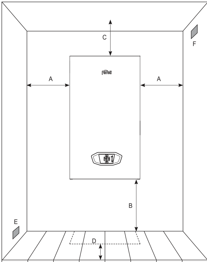
Рис. 3. Место установки
