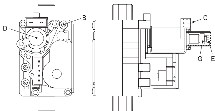
Рис. 12. Газовый клапан
