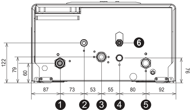
Рис. 4. Vitabel 10-24 кВт
