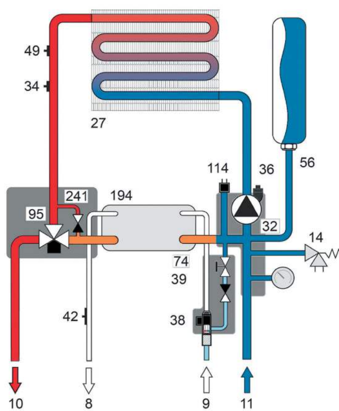
Рис. 14 Гидравлический контур
