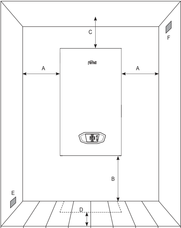
Рис. 3. Место установки
