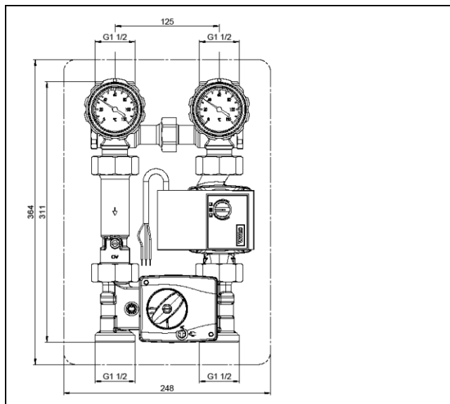
Рис. 4.3 „Regumat M4-130“ DN 25
