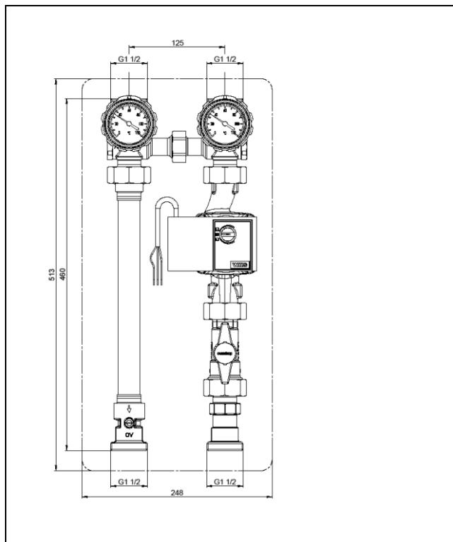
Рис. 4.7 „Regumat S-180°“ DN 25 с шаровым краном перед насосом
