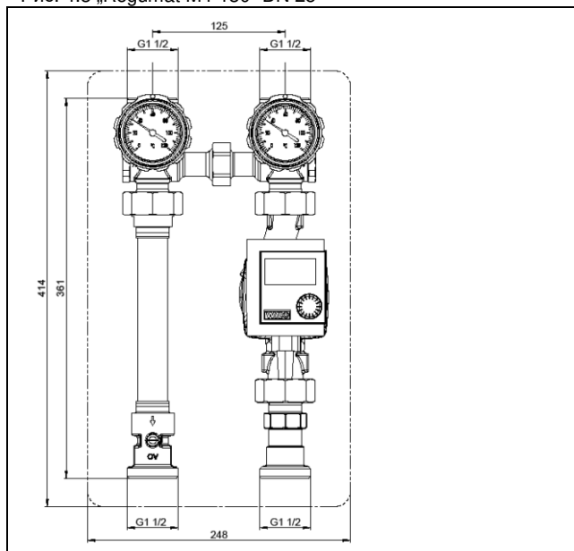
Рис. 4.4 „Regumat S-180“ DN 25
