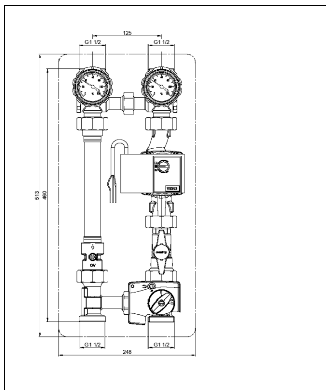
Рис. 4.8 „Regumat M3-180°“ DN 25 с шаровым краном перед насосом
