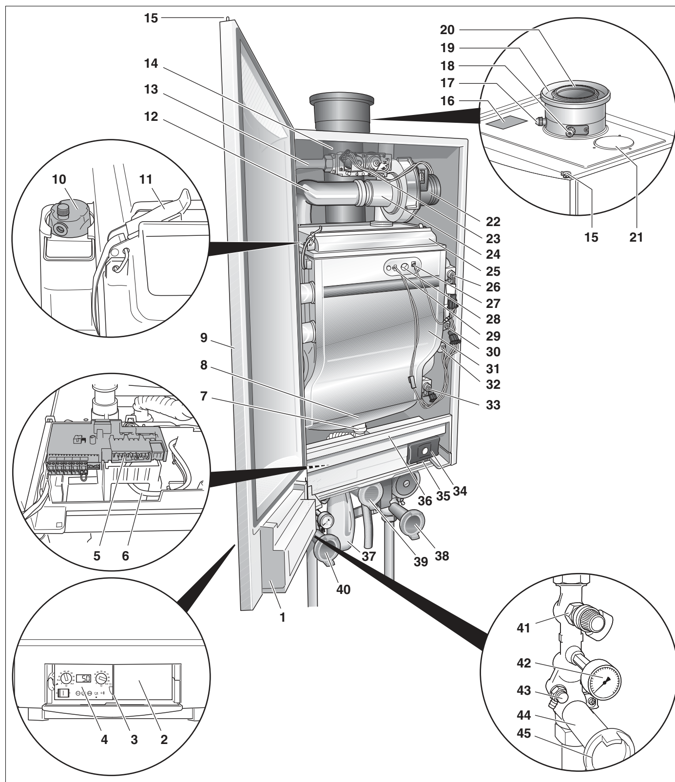
Рис. 1 Logamax plus GB162-65/80/100 с группой подключения
