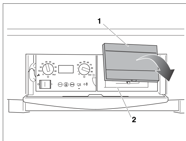
Рис. 29 Снятие заглушки и монтаж блока управления помещения RC35 на отопительном котле с функцией регулирования отопления по наружной температуре
