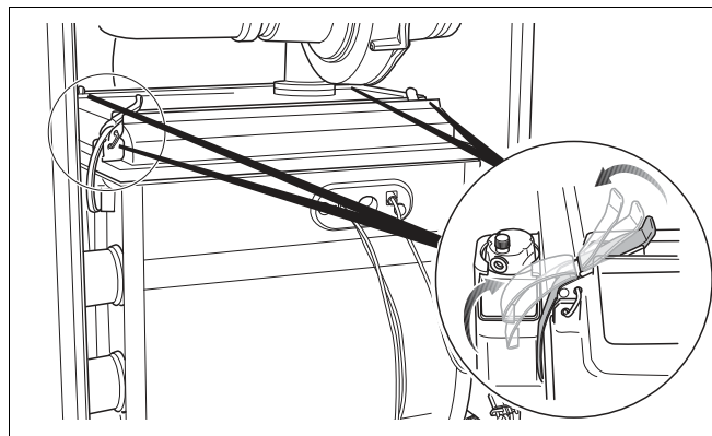
Рис. 103 Открывание защелок
