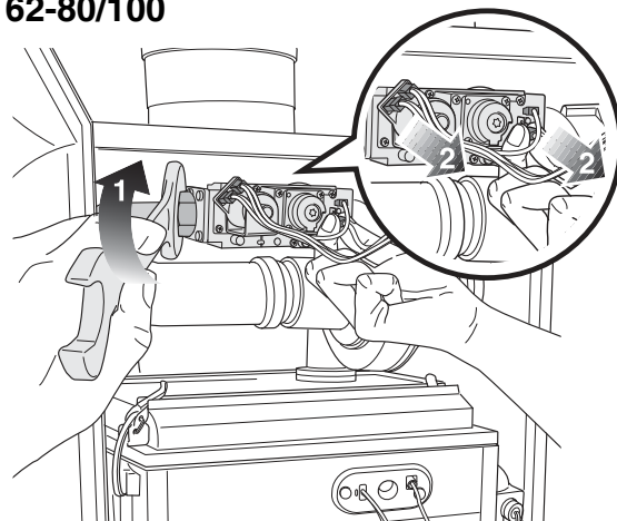
Рис. 100 Отсоединение подключений газовой арматуры
