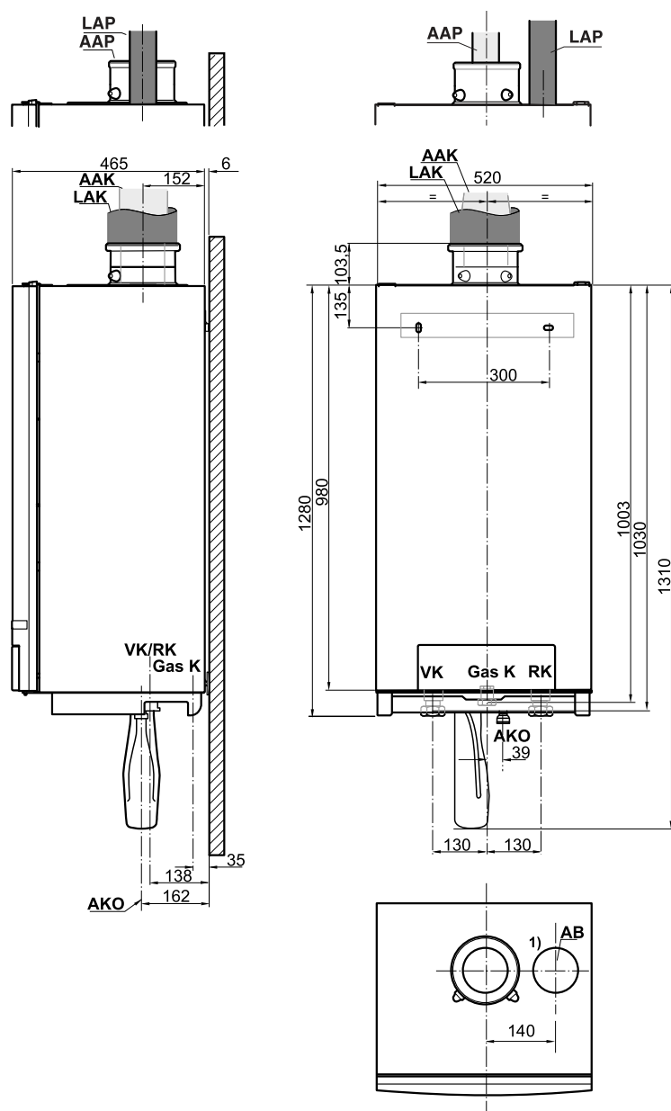
Рис. 5 Размеры и подключения без группы подключения (размеры в мм)
