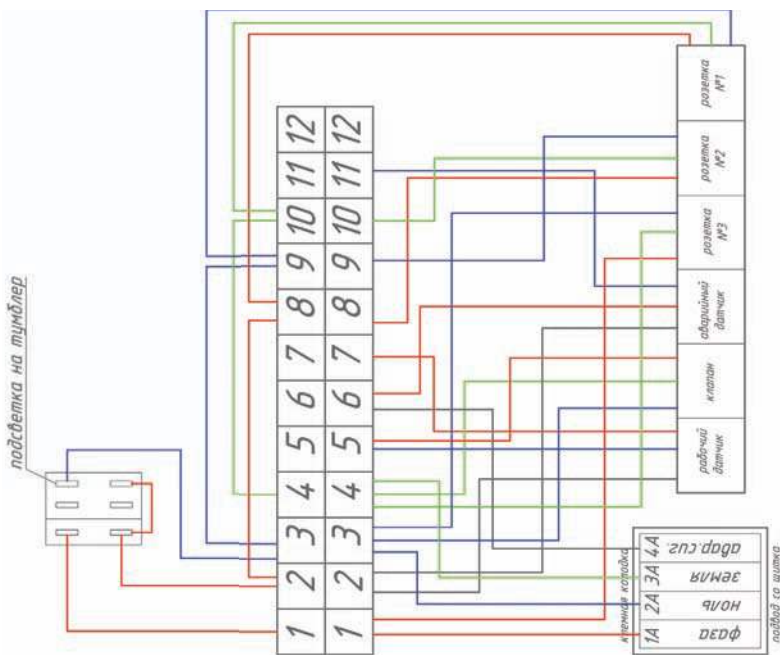
Схема распиайки клемной колодки с принудительным насосом ТОПАС 40-50
