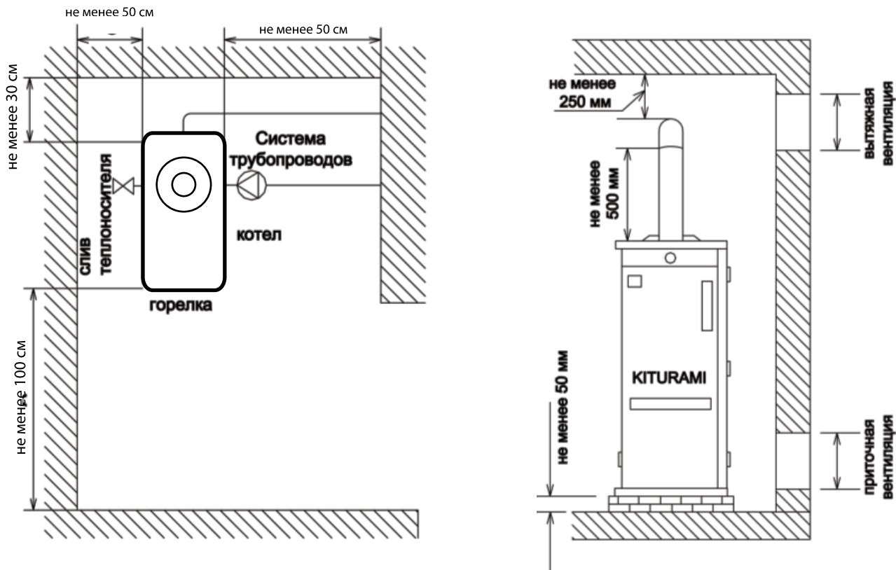
Рисунок 16. Установка котла
