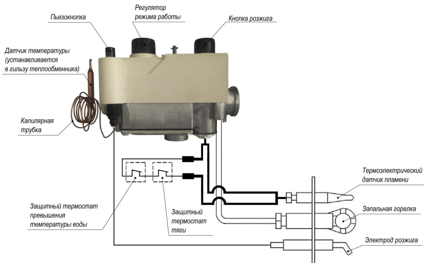
Рисунок 9. Схема соединений газового клапана.
