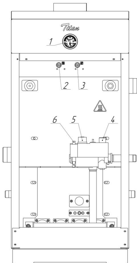
Рисунок 7. Расположение приборов управления котла
