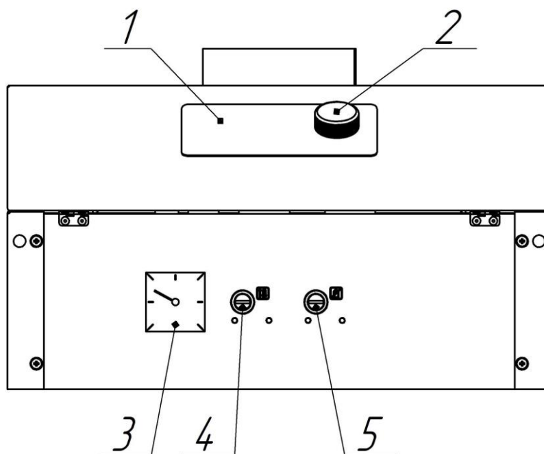
Рисунок 9. Расположение приборов управления котла (Вид показан при снятой передней панели котла)
