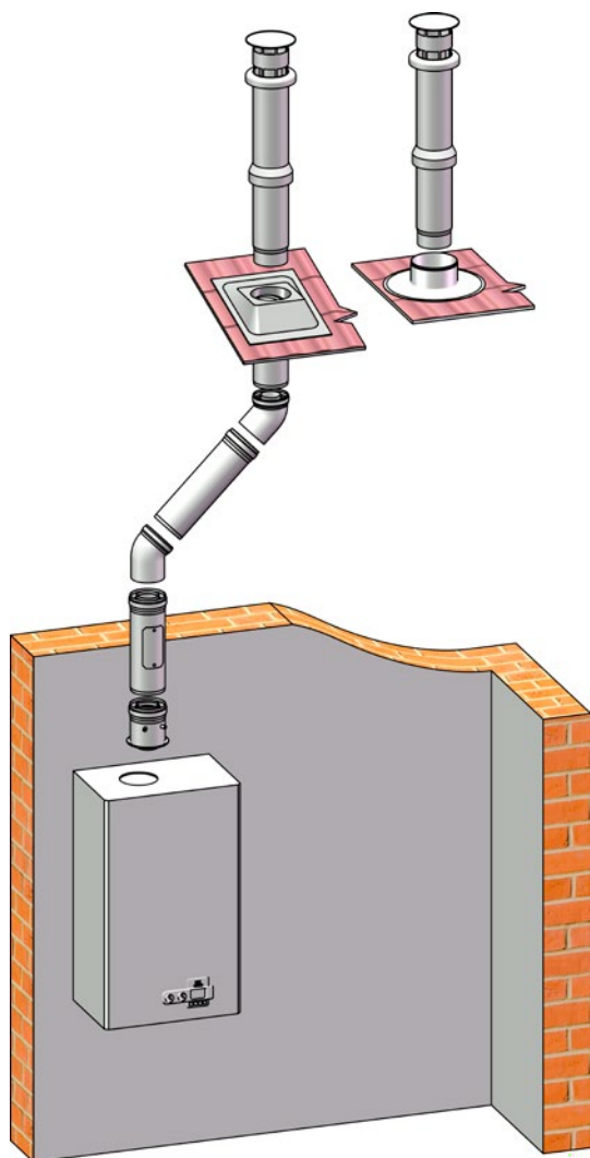
Коаксиальная система (60/100, 80/125)
