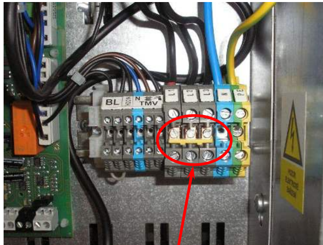
Подключение к однофазной сети эл. котла EL 5, EL 8, EL 9, EL 14
