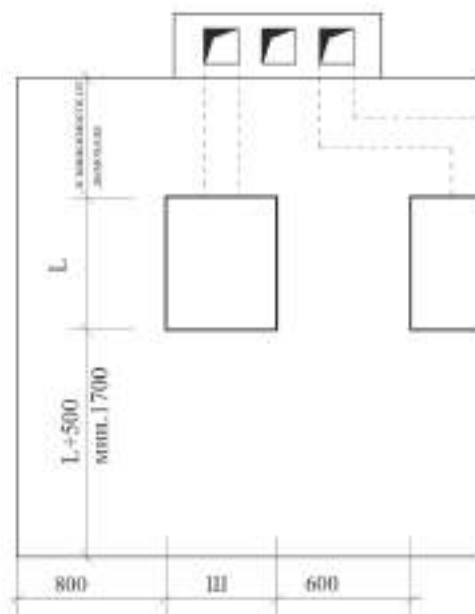
Рис. 7. Планировка котельной.
