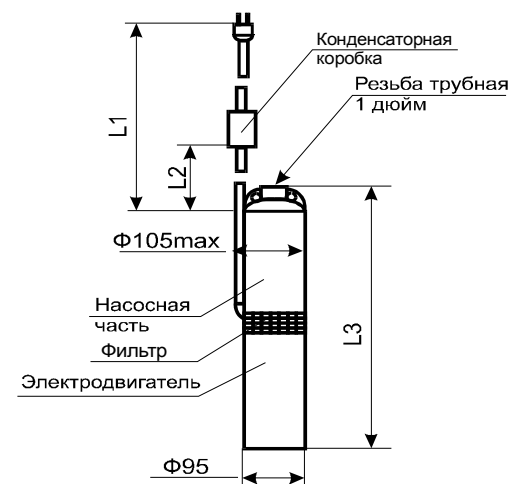
Габаритные и присоединительные размеры
