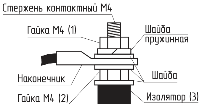
Рис.11 Присоединение проводов к выводам блок ТЭН
