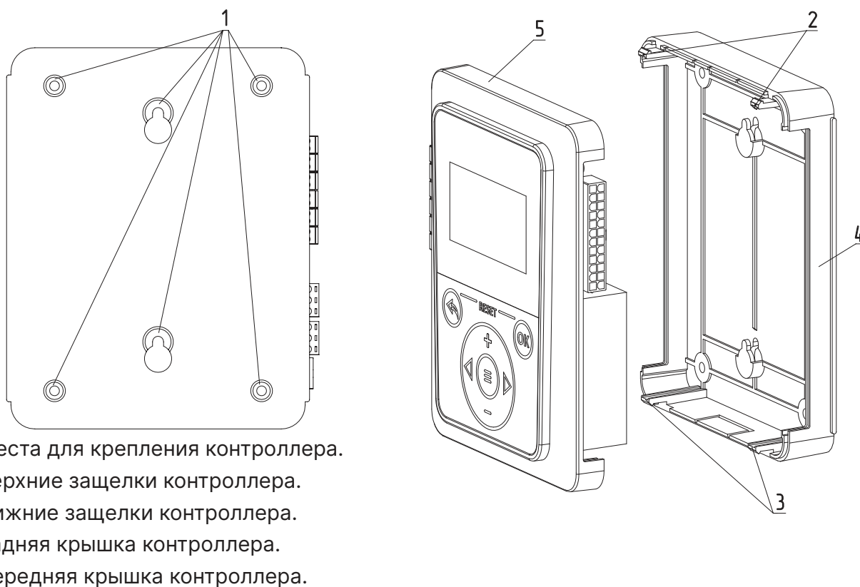
Рис.1 Корпус контроллера «ZOTA X-Line 100E»
