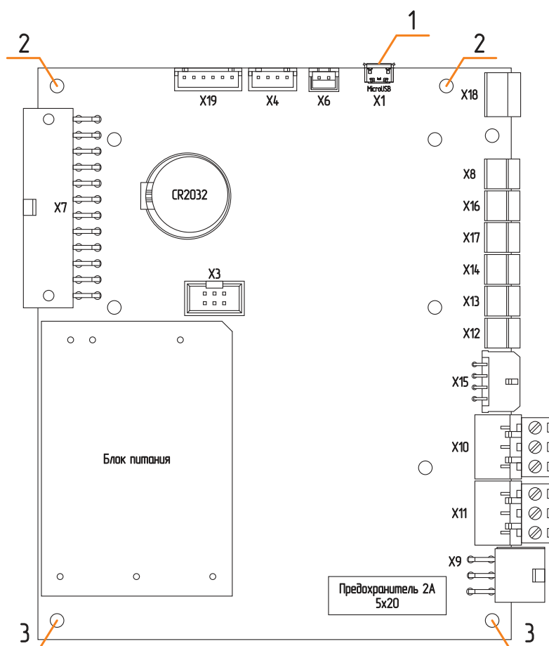
Рис.13 Плата контроллера
