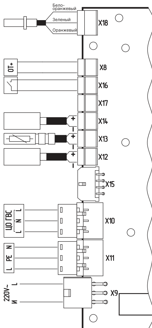
Рис.4 Схема подключения датчиков «ZOTA X-Line100E».
